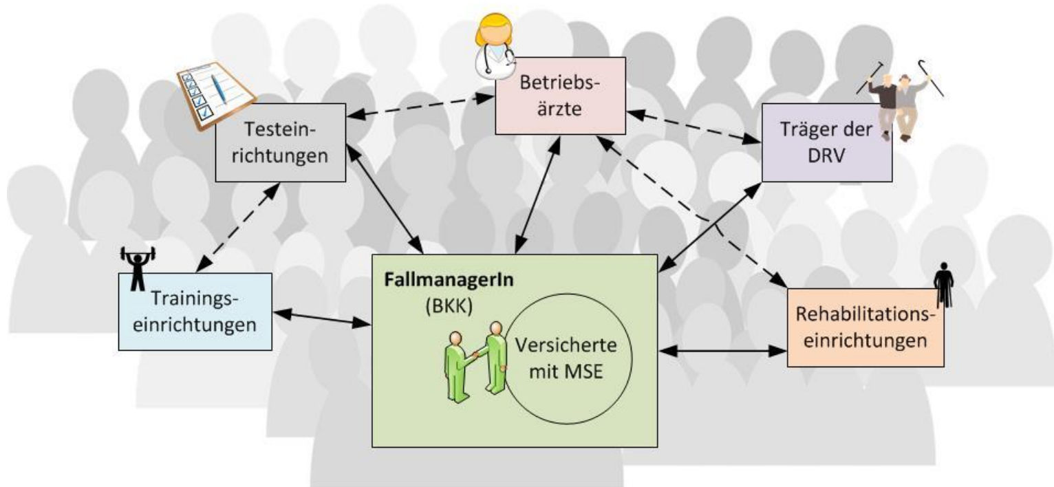
Abbildung 1: Versorgungsnetzwerk BGM-innovativ
