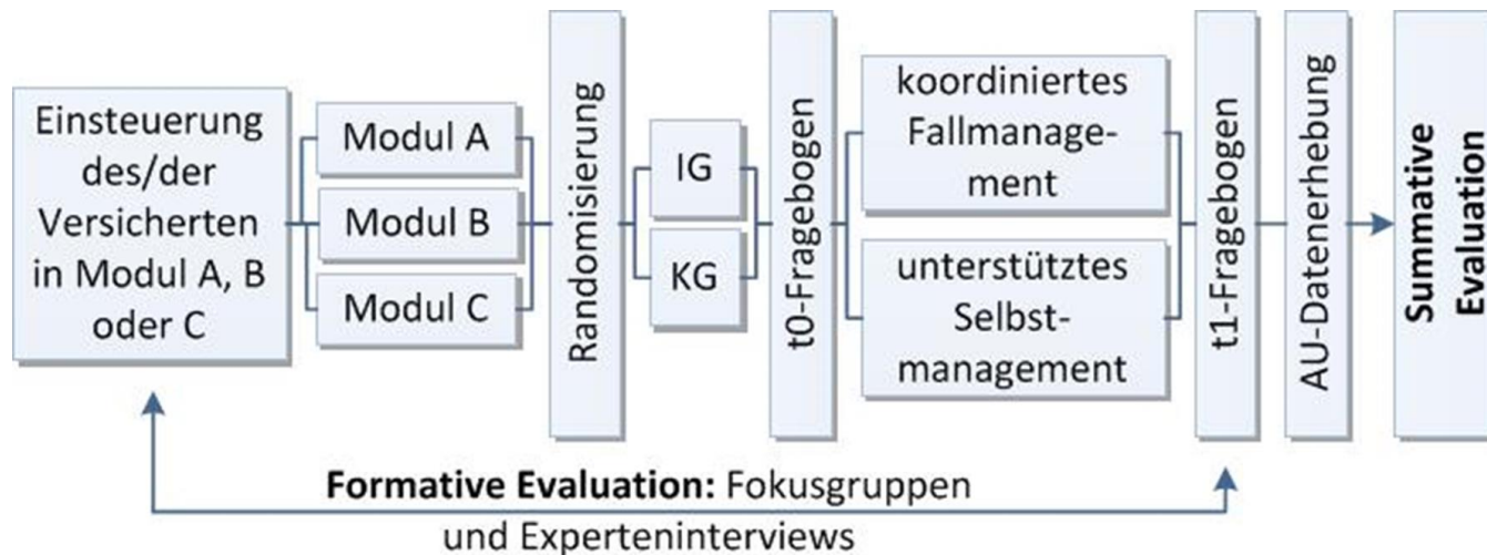
Abbildung 2: Evaluation BGM-innovativ
