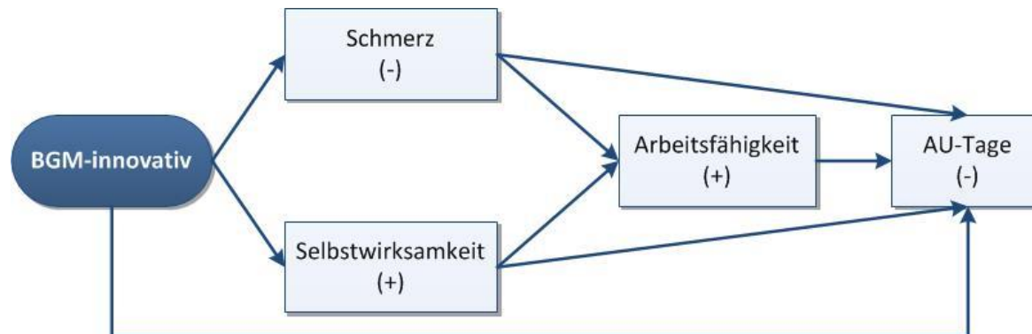
Abbildung 3: Wirkmodell BGM-innovativ
